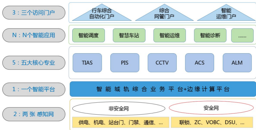
图 18 智能城轨一体化管控平台
