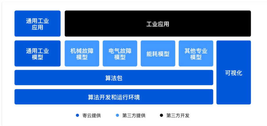
图 32 集成处理层架构图
