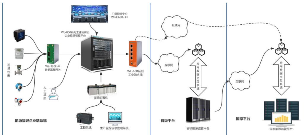
图 43 能源管理系统拓扑图
