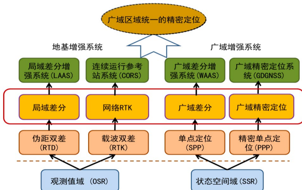
图 17 位置云服务广域区域统一的精密定位示意图
