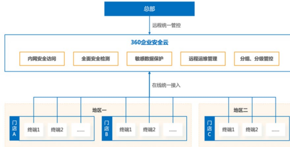
图 23 终端统一管理应用示意图
