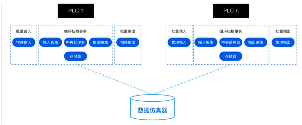
图 33 建模分析层架构图
