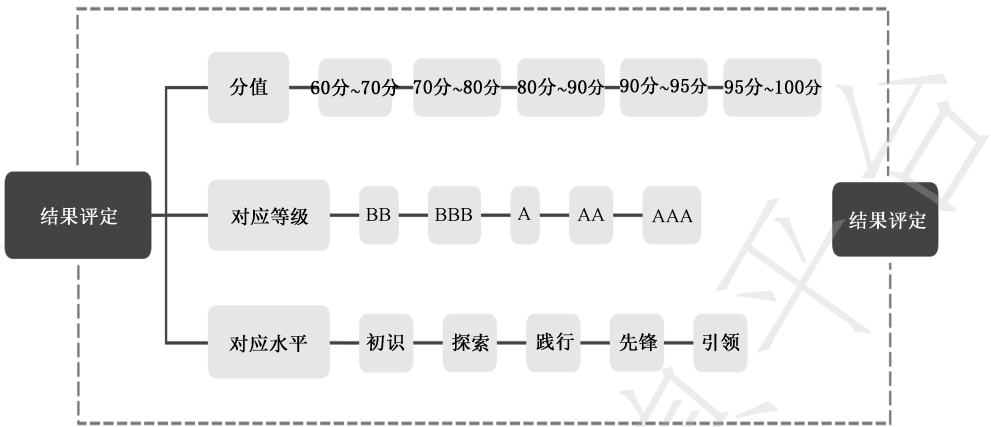
图 4 评价结果
