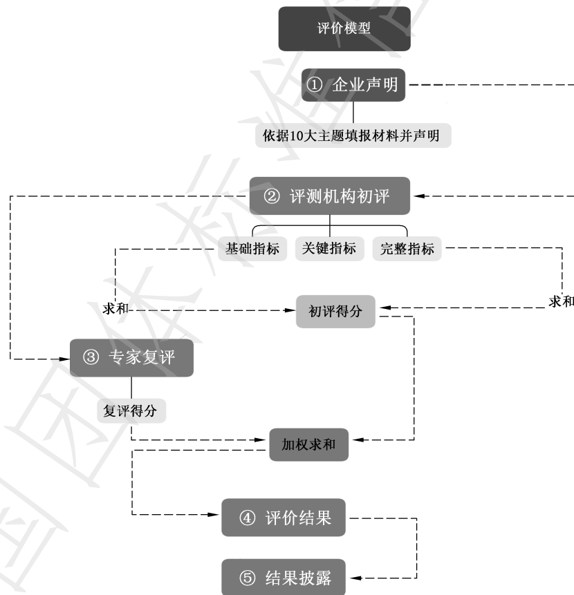
图 1 评价模型
