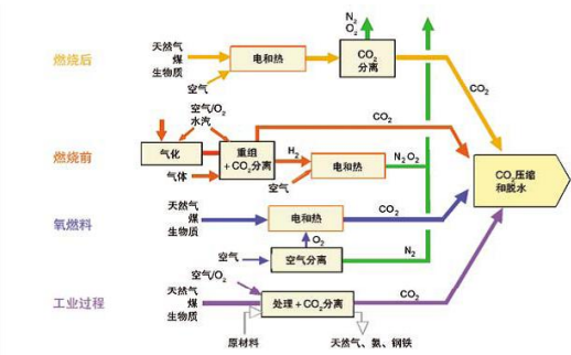
图 1 CO 2 捕获流程和系统概况
