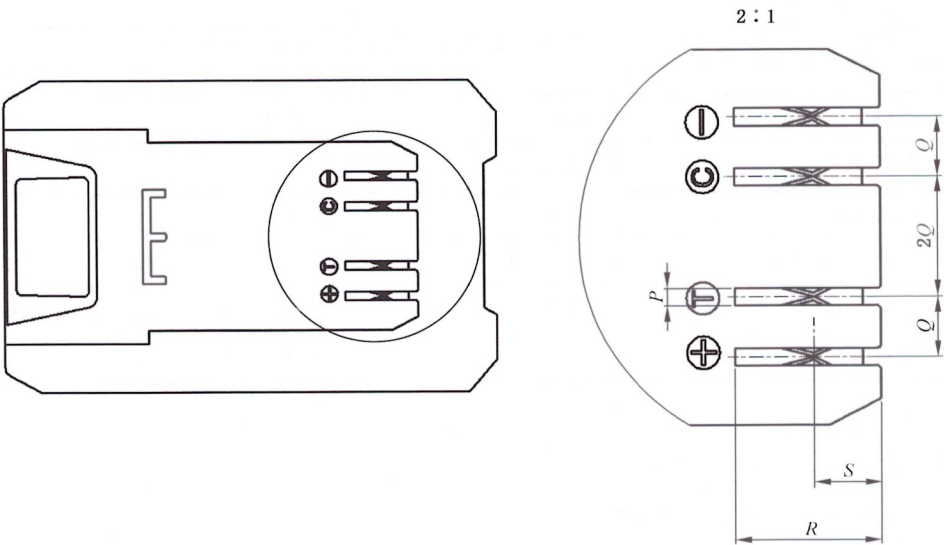
图 4 接口母插槽尺寸
