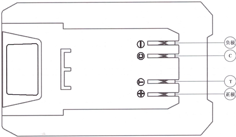
图 5 电池包接口端子
