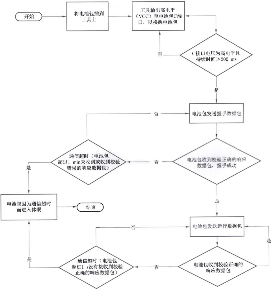
图 A.1 电池包与工具通信协议的执行逻辑
