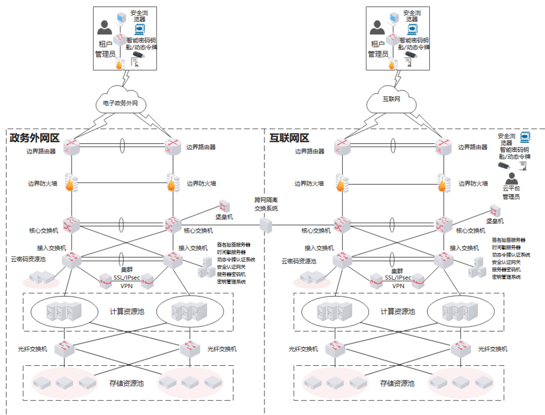
图 3 典型政务云平台密码应用部署图
