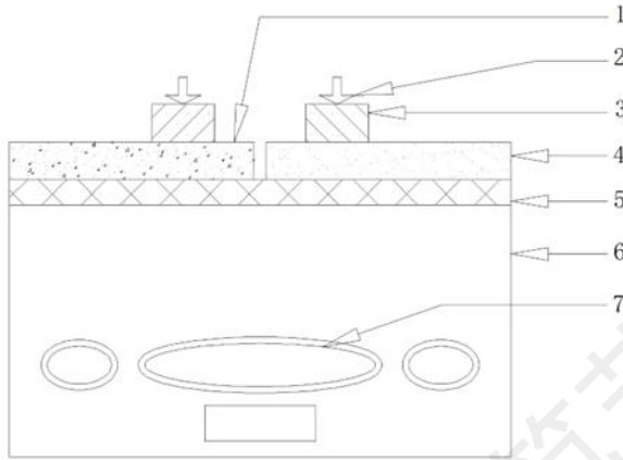
1-测试板；2-测温探头；3-高导热铝块；4-对比板；5-隔热垫； 6-测试箱体；7-热源（电阻加热器、磁管加热器、石墨烯加热片）
