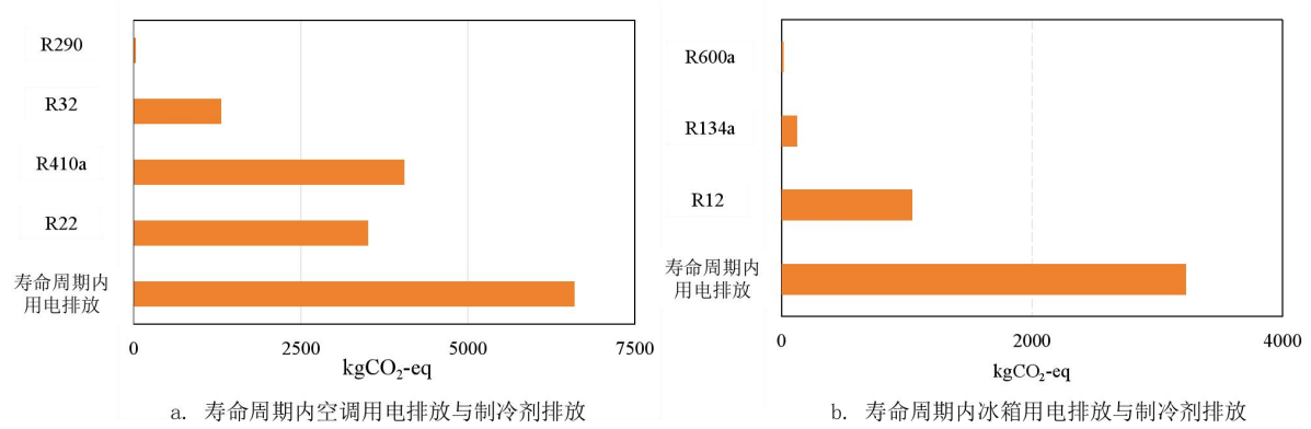
图 S1.3 寿命周期内设备制冷剂温室气体排放与用电排对比
