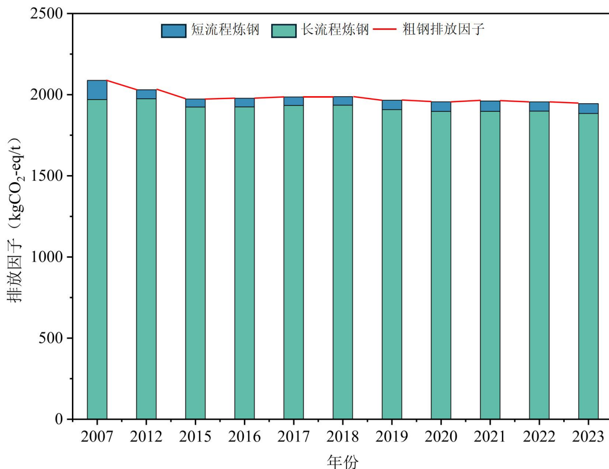
图 S2.4 2007-2023 年粗钢排放因子及排放结构
