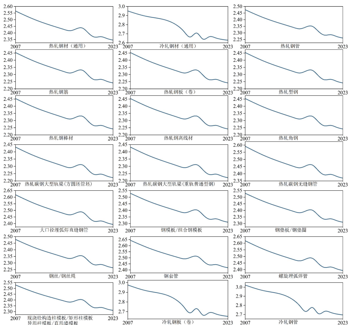
图 S2.5 2007-2023 年不同钢材排放因子 ( \text{t CO}_2\text{-eq/t} )
