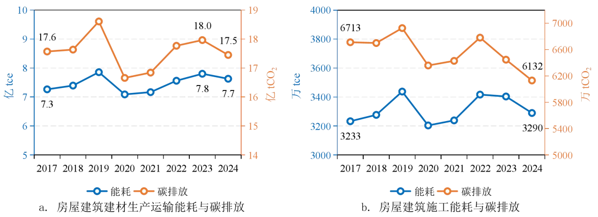
图 1.1 房屋建筑建造能耗与碳排放变化趋势
