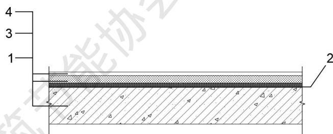
1-楼面基层（含找平层）；2-防水隔离层； 3-装配式保温隔声模块；4-饰面层
