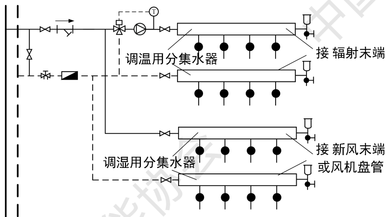
图 1 辐射末端和新风/风盘末端并联模式
