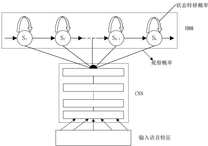
图 8-5 CNN-HMM 模型结构图
