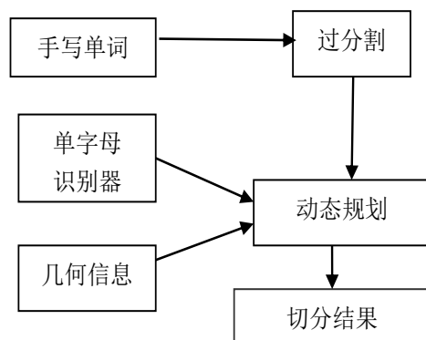
图 8-31 联机手写单词分割算法流程图
