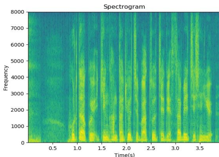
图 8-20 语谱图示例
