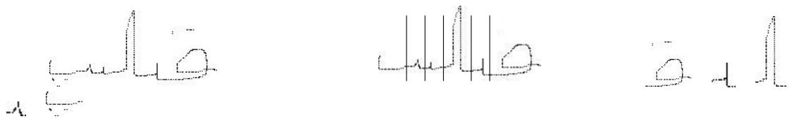
图 8-30 过切分结果
