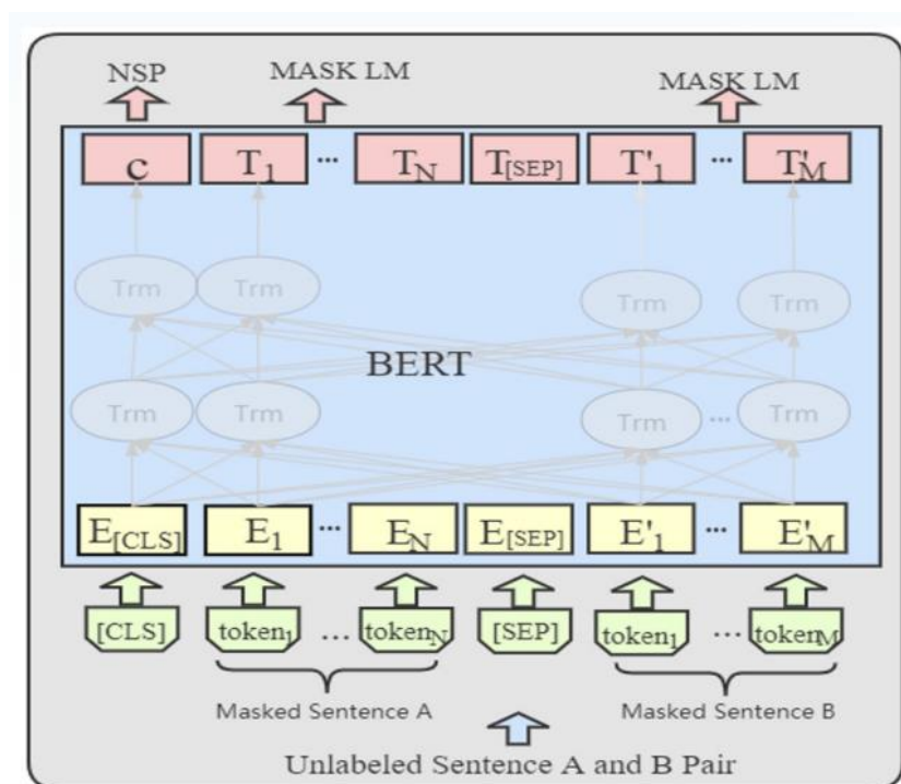
图 5-1 BERT 模型
