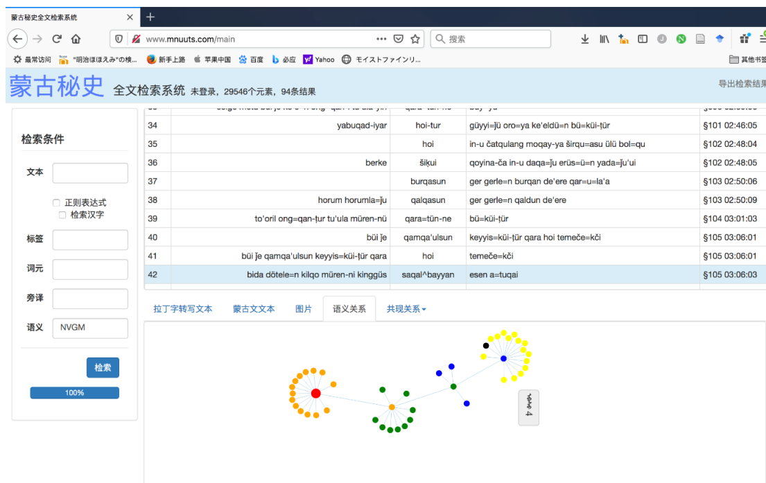
图 2-9 语义检索
