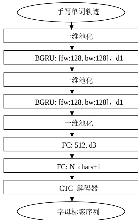
图 8-36 RNN-CTC 无约束联机手写维吾尔文单词识别模型结构
