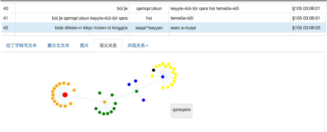
图 2-10 语义关系
