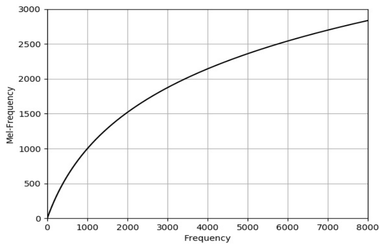
图 8-17 Mel 频率图
