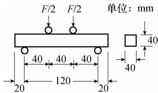
图 A.1 三等分抗折强度试验示意
