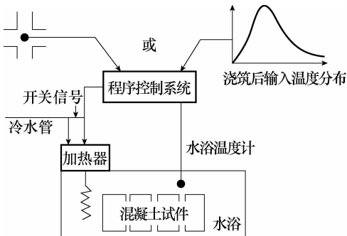
图 B.1 温度跟踪养护装置示意
