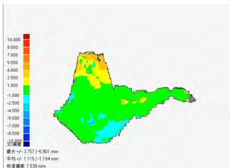
图5 色谱分析
