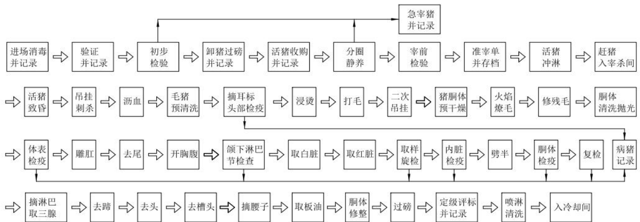
图 1 生猪屠宰工艺流程
