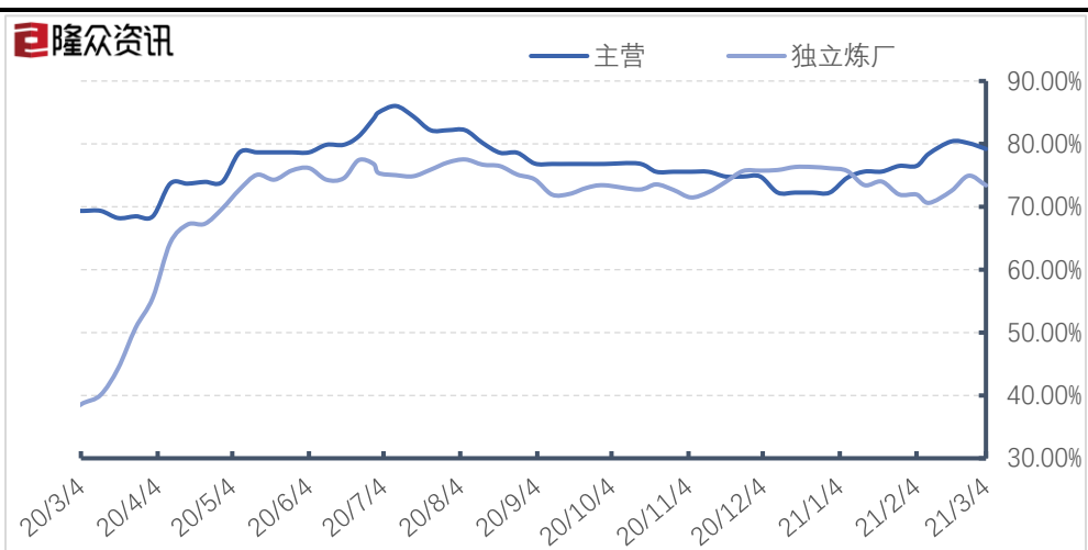
图 2 中国主营及独立炼厂常减压装置利用率走势图
