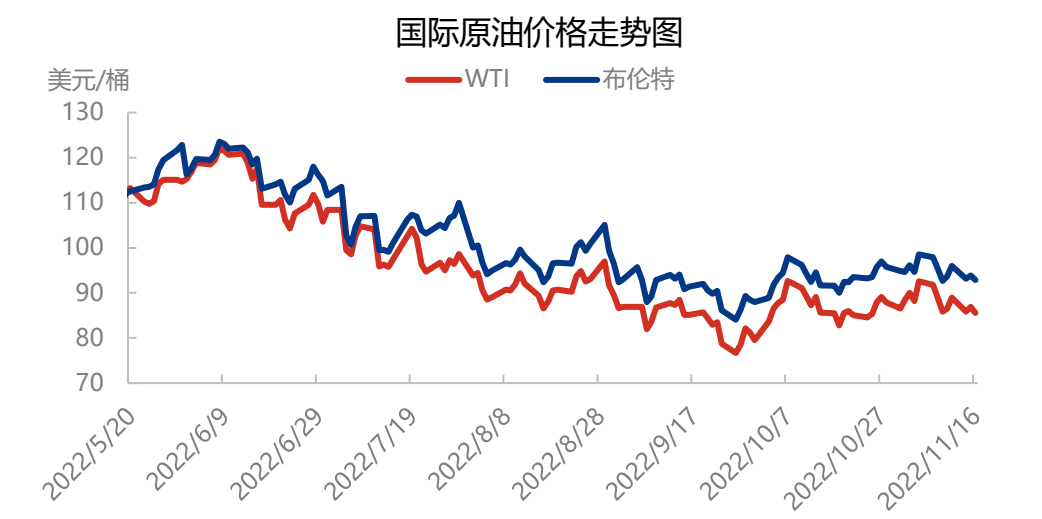
图表 5 国际原油价格走势
